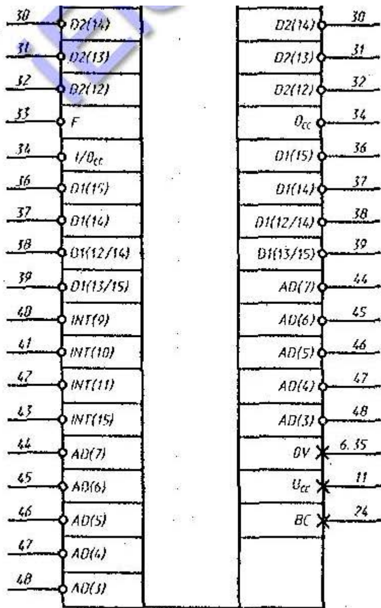
Условное графическое обозначение 1827BE1 K1827BE1
